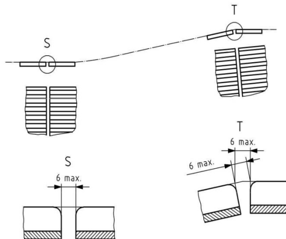
شکل ۶- شمائی از صفحات حمل کننده، فاصله آزاد و عمق شبکه (پیاده‌روهای متحرک صفحه‌ای بدون لبه‌های جلویی و کناره‌های عقبی مشبک) در انحنای گذار و محل سوار و پیاده شدن‌های بالائی و پائینی (ابعاد بر حسب میلی‌متر)
