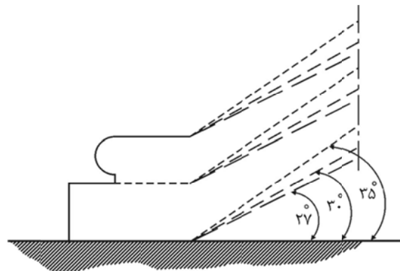
شکل ۱۱-۱-۳-۱۵ زوایای شیب پلکان برقی
