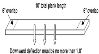
امتداد تخته‌ها در انتهای داربست جهت ایجاد تکیه گاه مناسب
